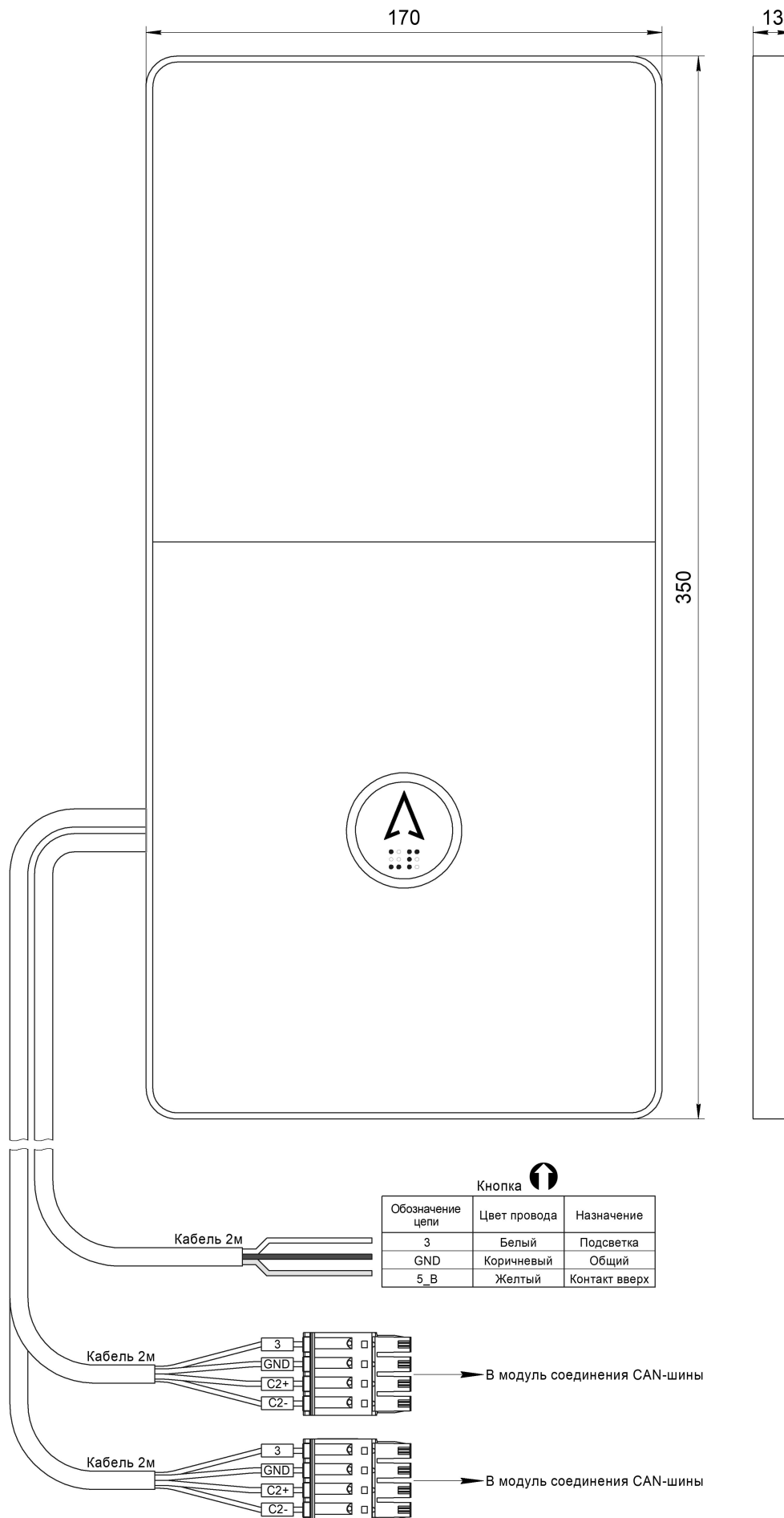
Рис.1 Внешний вид, габаритные и установочные размеры Вызывного поста МАЛАХИТ НШЕК.468381.017
